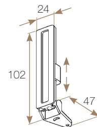
POULIE DE BAS , polyamide Poulie montée sur axe acier, convient pour les cordons \varnothing 3,5 à 4 mm. Fixation par 2 vis apparentes F \varnothing 4 mm (vis de pose non fournies).
