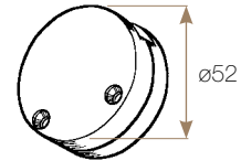
POULIE DE BAS , polyamide Poulie montée sur axe acier, convient pour les cordons \varnothing 3,5 à 4 mm. Fixation par 2 vis apparentes F \varnothing 4 mm (vis de pose non fournies).
