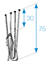
AGRAFE 4 BROCHES , acier zingué fil ø2 mm.
