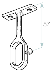
SUPPORT DE PENDERIE , alliage Pour tube ovale 30x15 mm. Fixation par 2 vis apparentes F \varnothing 5 mm (vis de pose non fournies). Coloris : chromé.
