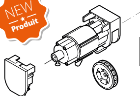
ENSEMBLE MÉCANISME AVEC SÉCURITÉ ENFANT , plastique.
