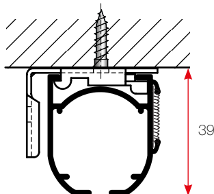
Pose au plafond avec support universel
