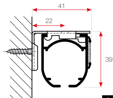
Pose au mur ou sur fenêtre avec support universel - Retour 2 cm
