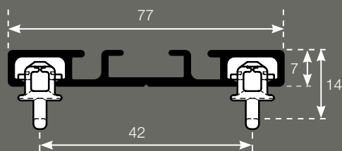
Pose directe au plafond : 2 voies avec voilages
