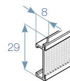
RAIL PORTE-TOILE 29X8 MM, Aluminium blanc avec galon crochet. Longueur : 3M00
