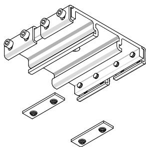
MANCHON , Aluminium Pour 2 rails. Fixation par 1 vis ø8 mm (vis de pose non fournies).
