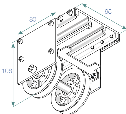
POULIE DE TIRAGE , Aluminium avec sa fixation pour pose directe plafond. Fixation par 2 vis ø8 mm (vis de pose non fournies).
