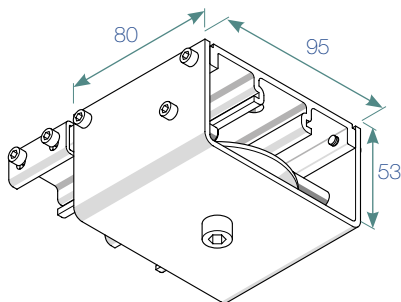
POULIE DE RENVOI , Aluminium avec sa fixation pour pose directe plafond. Fixation par 2 vis ø8 mm (vis de pose non fournies).
