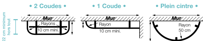
Cintrage extérieur
