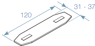
RACCORD , Acier zingué. Pour 2 et 3 voies : 31x120x2 mm Pour 4 et 5 voies : 37x120x2 mm S'utilise pour raccorder deux rails.
