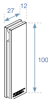
POULIE LESTÉE , Acier et plastique Pour cordon de \varnothing 3 à \varnothing 3,5 mm. Poids : 110 gr
