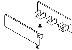
PAIRE D'EMBOUITS POUR RAIL 3 VOIES, Plastique blanc. Avec vis de blocage.
