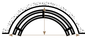
Plein cintre
