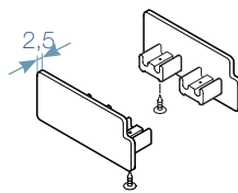
PAIRE D'EMBOUITS POUR RAIL 2 VOIES, Plastique blanc. Avec vis de blocage.
