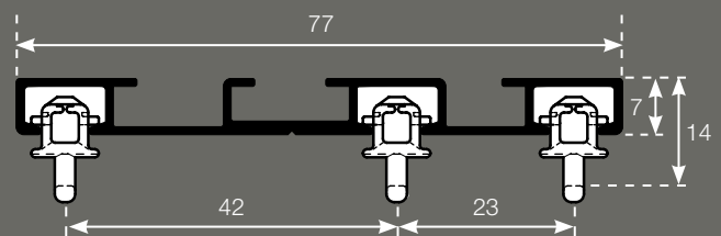
Pose directe au plafond : 3 voies avec voilages
