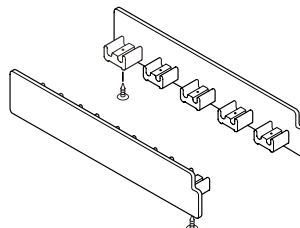
PAIRE D'EMBOUITS POUR RAIL 5 VOIES, Plastique blanc. Avec vis de blocage.
