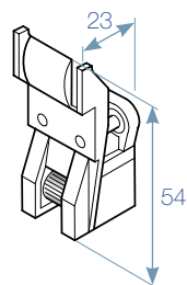
POULIAGE CORDONS , Plastique blanc, Auto bloquant. Pour cordon \varnothing 1,5 mm. Pour arrêter le store à la hauteur désirée.
