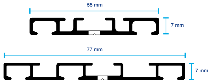
Rail plat 2 voies 7x55 mm et rail plat 3 voies 7x77 mm
