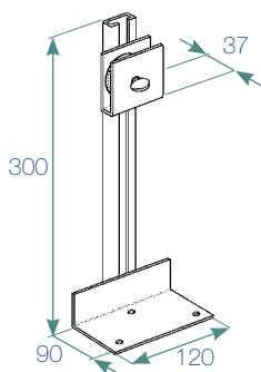
POULIE DE BAS TENDEUR , Acier Fixation par 3 vis apparentes ø6 mm (vis de pose non fournies).
