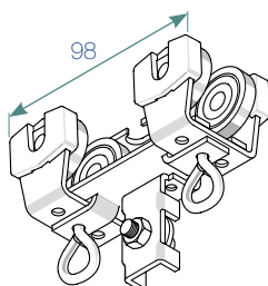
CONDUCTEUR , polyamide et acier Galets à billes montés sur axe acier.
