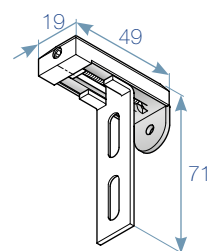
SUPPORT FENÊTRE PVC , Acier et plastique Ce support ne nécessite aucun perçage et se pose sur le haut de l'ouvrant de la fenêtre.
