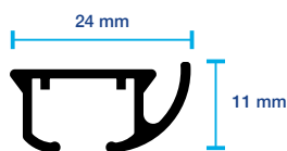
Rail DS - 24x11 mm
