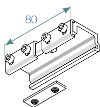
1/2 MANCHON , Aluminium Pour rail simple. Fixation par 1 vis ø8 mm (vis de pose non fournies).
