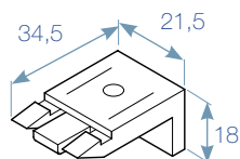
SUPPORT UNIVERSEL , Plastique blanc Pour poses au plafond ou au mur des mécanismes à cordons.
