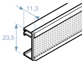
RAIL 23,5x11,3 mm , Aluminium blanc avec galon crochet. Longueur minimum : 35 cm Longueur max : 6M00
